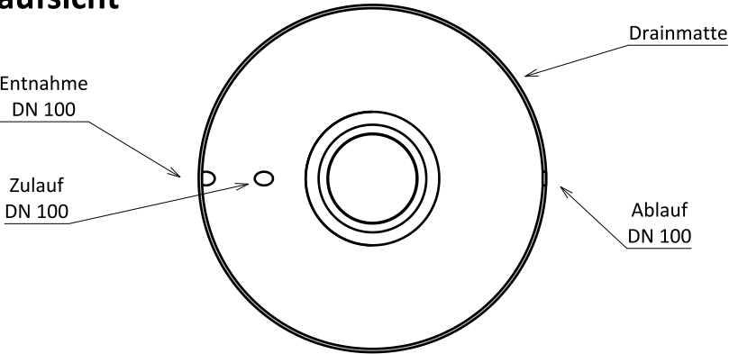
Draufsicht
